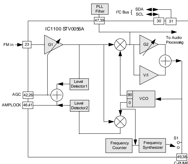
Blockschaltbild Audio-Demodulator
